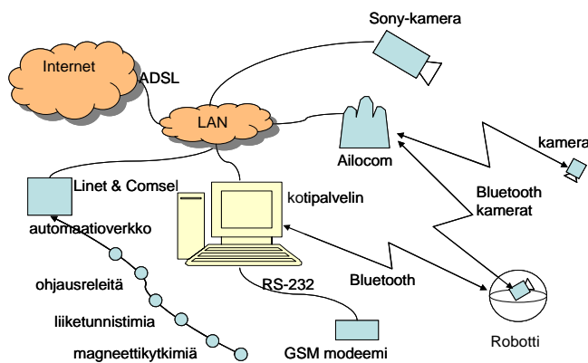
Kuva 9. Toteutetun kotiautomaatiojärjestelmän yleiskuva
