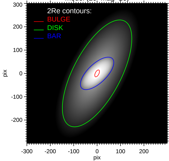
model (20&lt;mag&lt;26)
